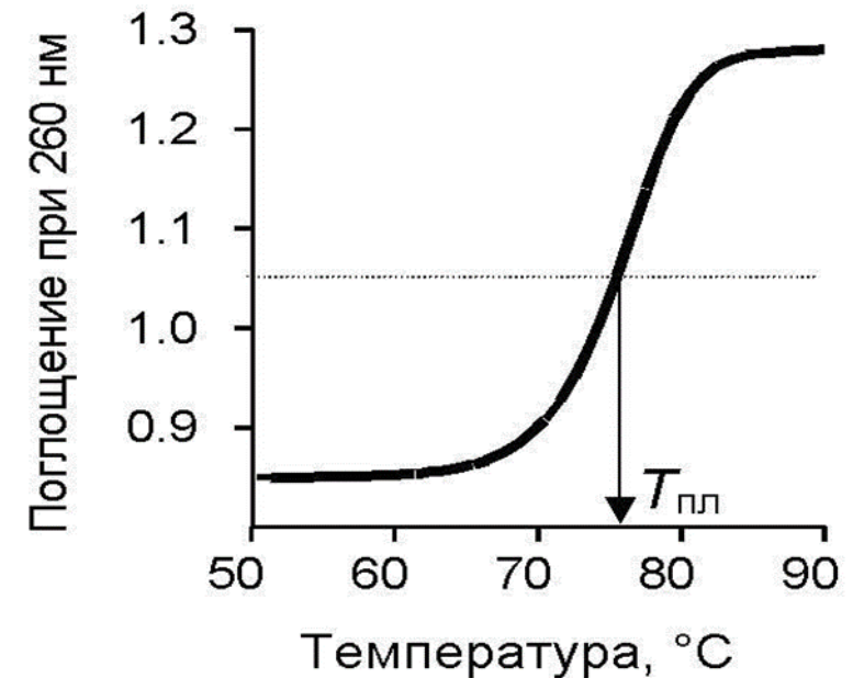
ДНК балқу қисығы
